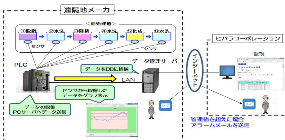
図2-3-4 前処理槽センシングシステム
