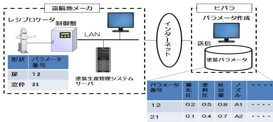
図2-3-3 遠隔工場での塗装機とPCの連動
